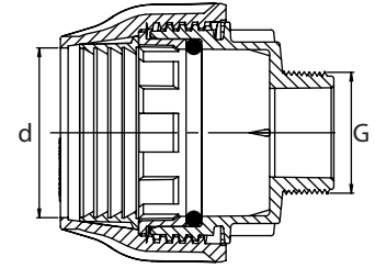
KABLİN ERKEK MALE ADAPTOR МУФТА С НАРУЖНОЙ РЕЗЬБОЙ بداية سن خارج
