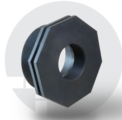
DIŞLİ REDÜKSİYON ERKEK - DIŞI THREADED REDUCING MALE - FEMALE BUSHING ПЕРЕХОДНИК РЕЗЬБОВОЙ «МУФТА» بوش مصغرة مسننة سن خارج - سن داخل
