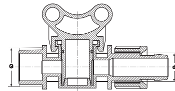
MİNİ VANA ERKEK - DAMLAMA MINI VALVE MALE - DRIPLINE МИНИ-КРАН «ШТУЦЕР» – ДЛЯ ТРУБЫ КАПЕЛЬНОГО ПОЛИВА قفل صغير سن خارج - تقطير
