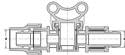
MİNİ VANA KİLİTLİ BAĞLANTI - DAMLAMA MINI VALVE LOCK TYPE - DRIPLINE МИНИ-КРАН С ЗАМКОМ – ТРУБА ДЛЯ КАПЕЛЬНОГО ПОЛИВА قفل صغير نوعية اففال - تقطير
